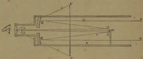
Fig. 189.—Gregorian Reflector.
