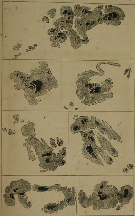
SUN-SPOTS. (Sir J. Herschel.)
