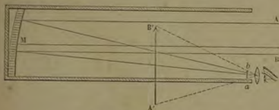
Fig. 190.—'Front View' Reflector.
