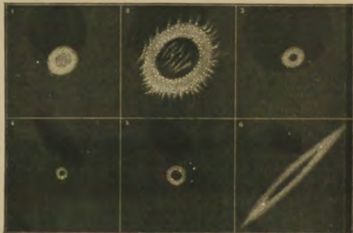
Fig. 152.—Annular Nebulae.
